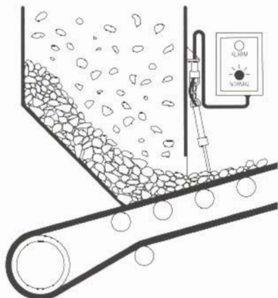
► Produktstroom detectie
